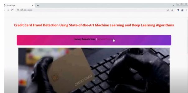
Fig.2. Login page.
