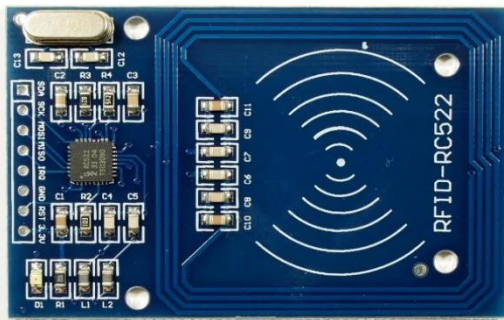
Fig 5: RFID Module
