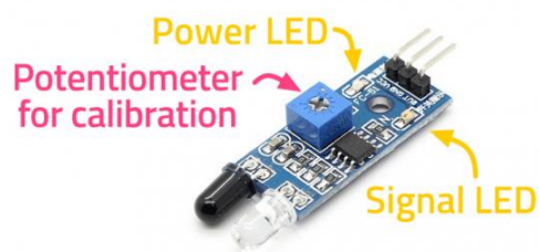
Fig 4: IR Module
